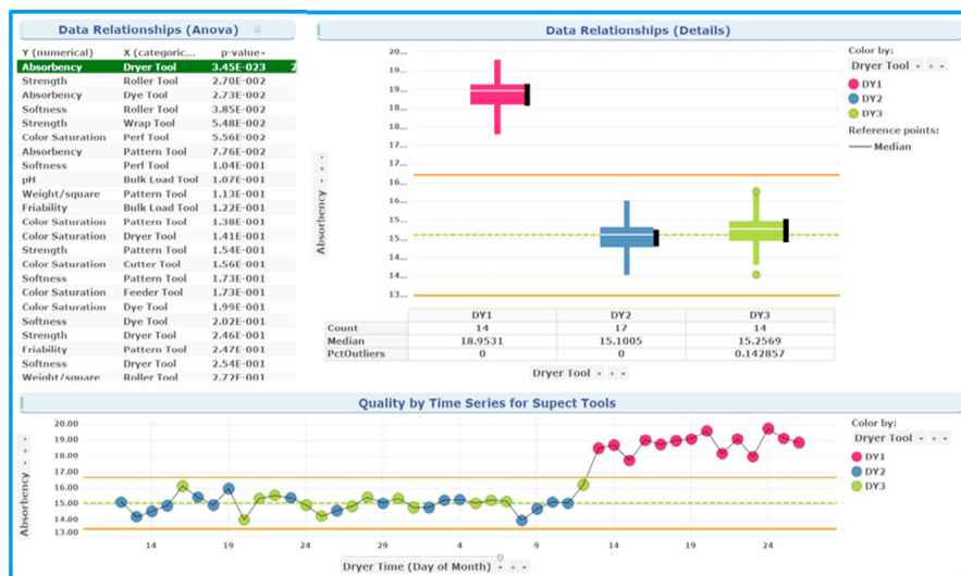
Figura 5.16 – Statistica .
