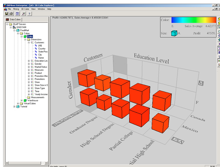
Figura 5.15 - DBMiner.
